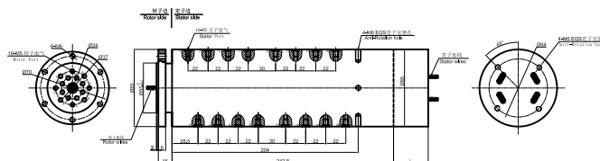
MAPH1600-01 尺寸图
